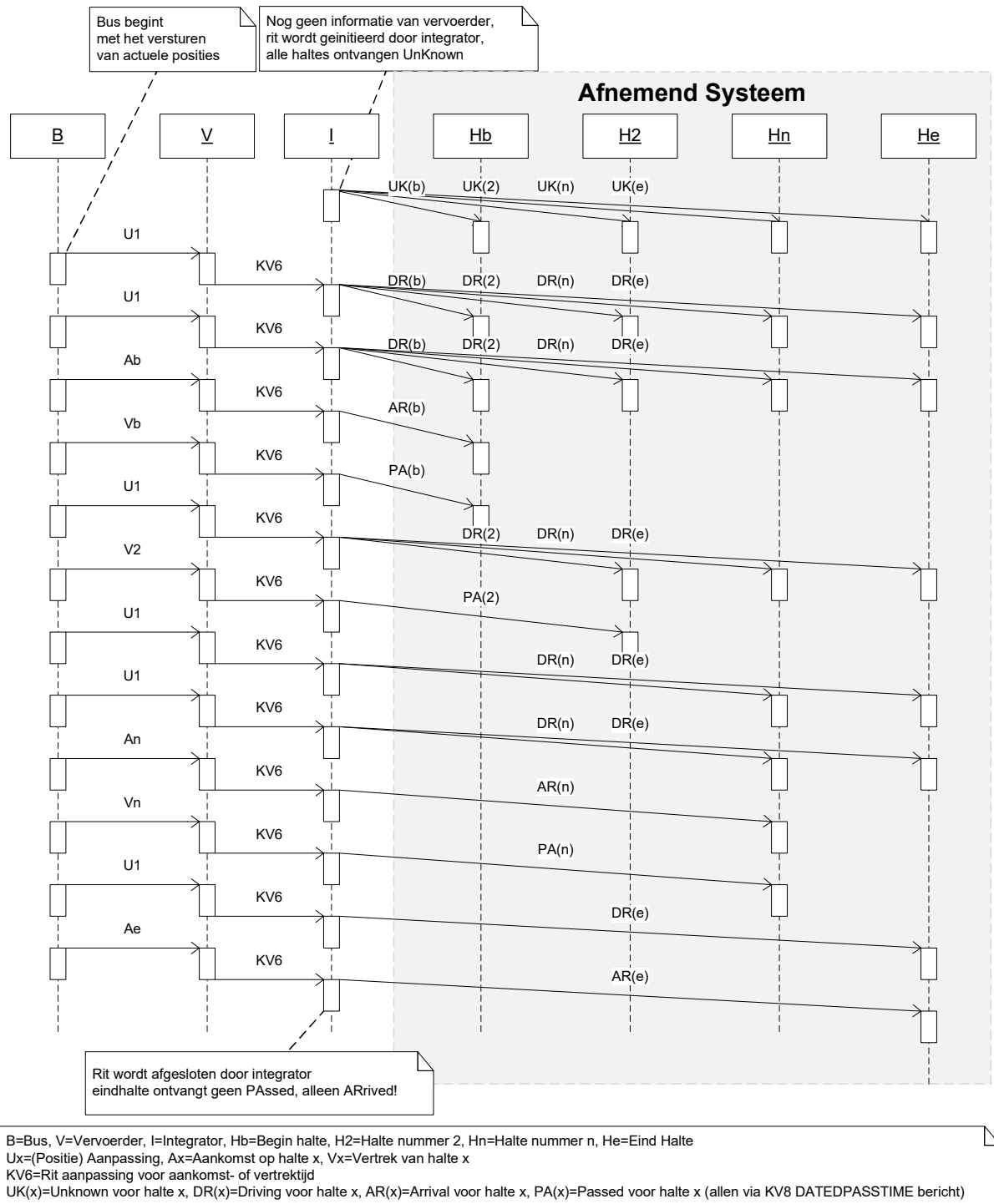
Figuur 6 Standaard Rit (Integratie Model)
