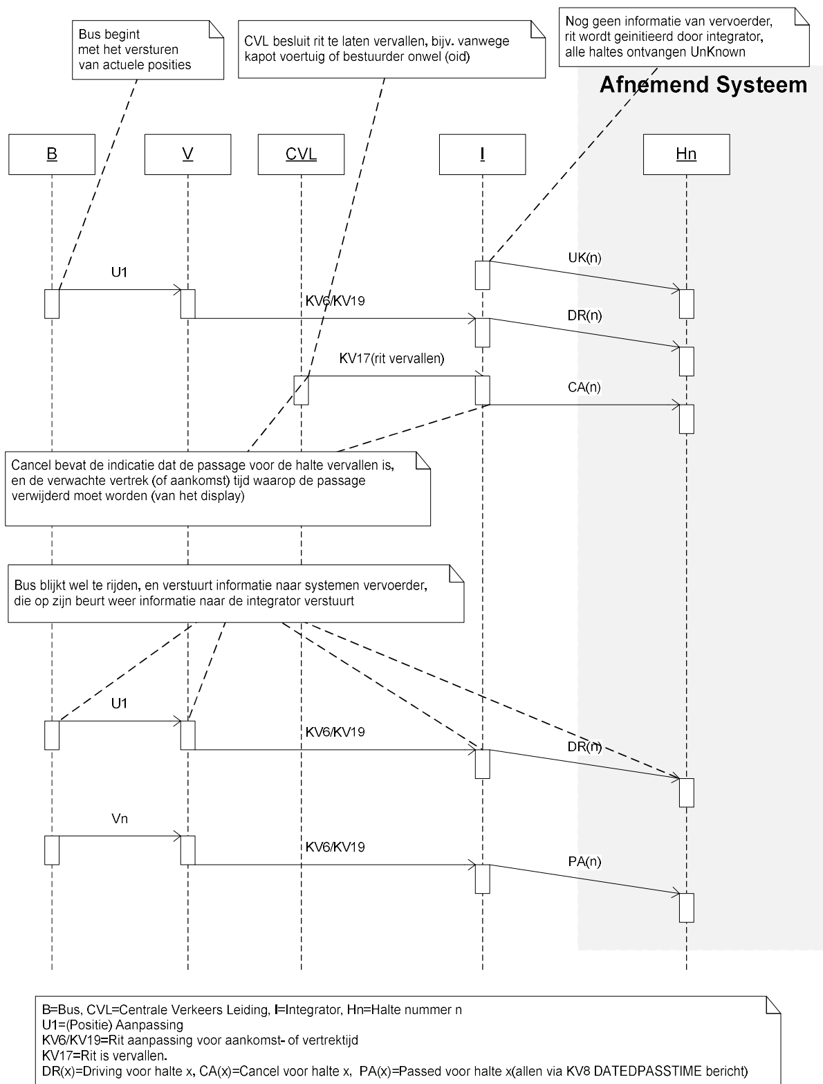
Figuur 10 Rit vervallen gedurende de rit uitvoering blijkt toch te rijden
