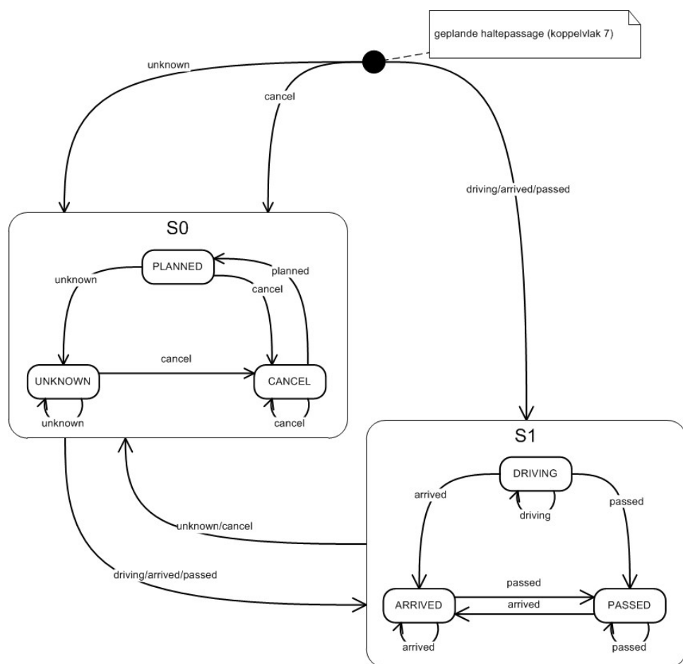
Figuur 5 TripStopStatus toestandsovergangen binnen S0 en S1
