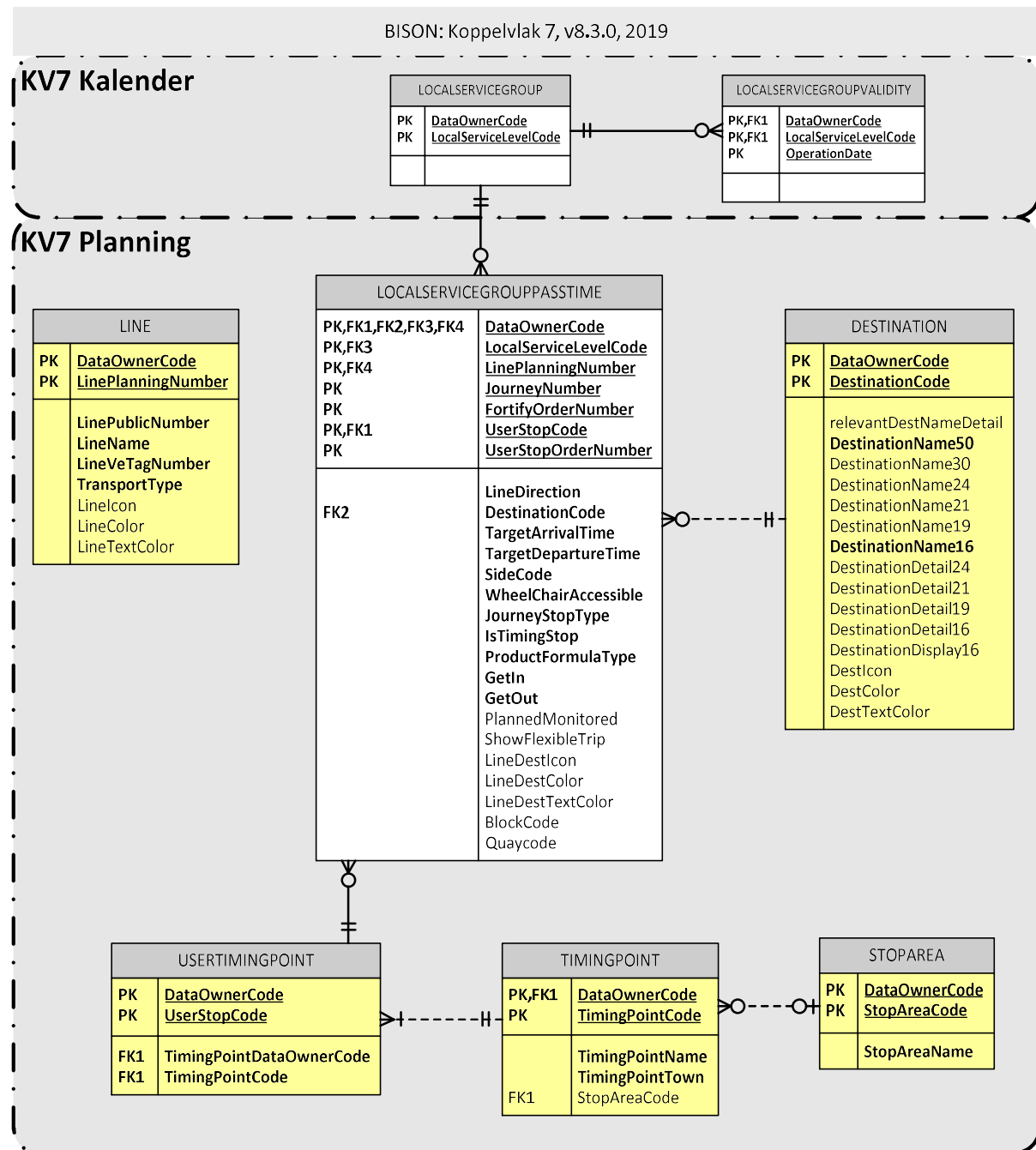
Figuur 2 Koppelvlak 7 Entity Relation Diagram
