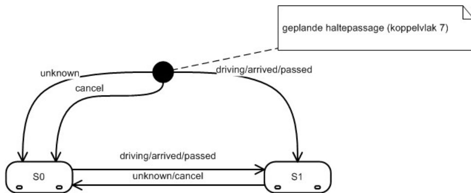
Figuur 4 TripStopStatus toestandsovergangen voor een passage
