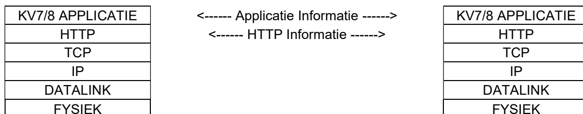
Figuur 34 Koppelvlak protocol stapel
