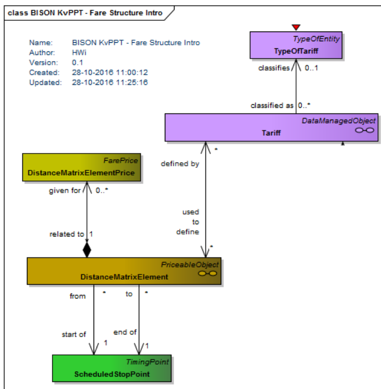
Figuur 18 UML, fysiek, Tariff met matrix
