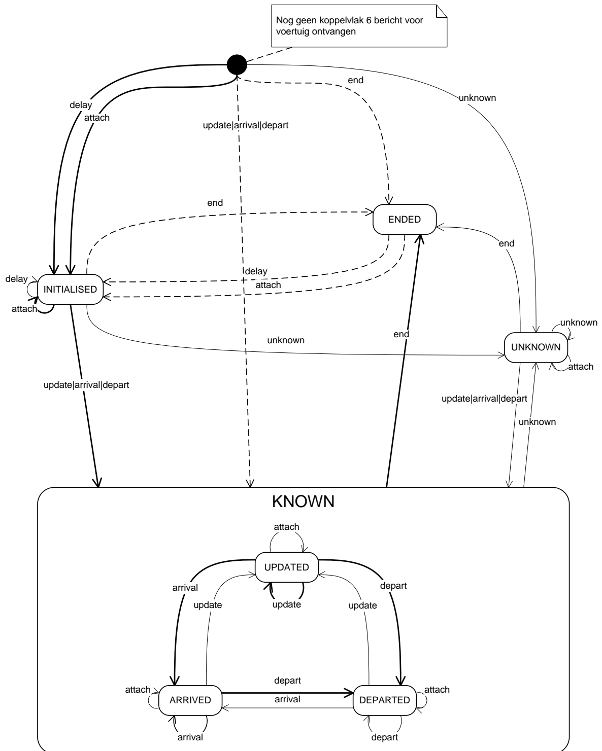
Figuur 38 Uitgebreid transitiediagram koppelvlak 6 berichten
