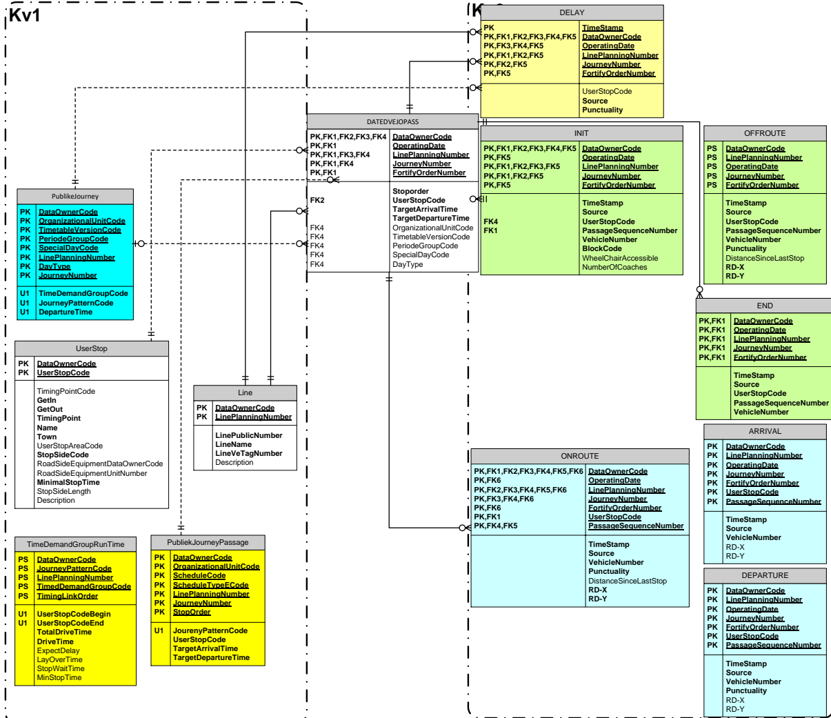
Figuur 35 Mogelijk gebruik van een DATEDVEJOPASS tabel tussen kv1 en kv6
