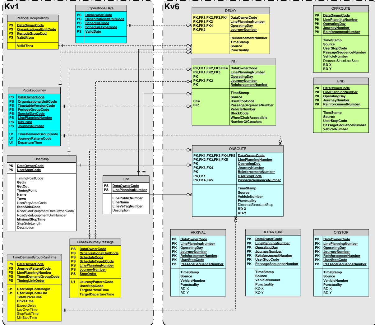
Figuur 34 Koppelvlak 6 ERD, relaties tussen Koppelvlak 6 en koppelvlak 1
