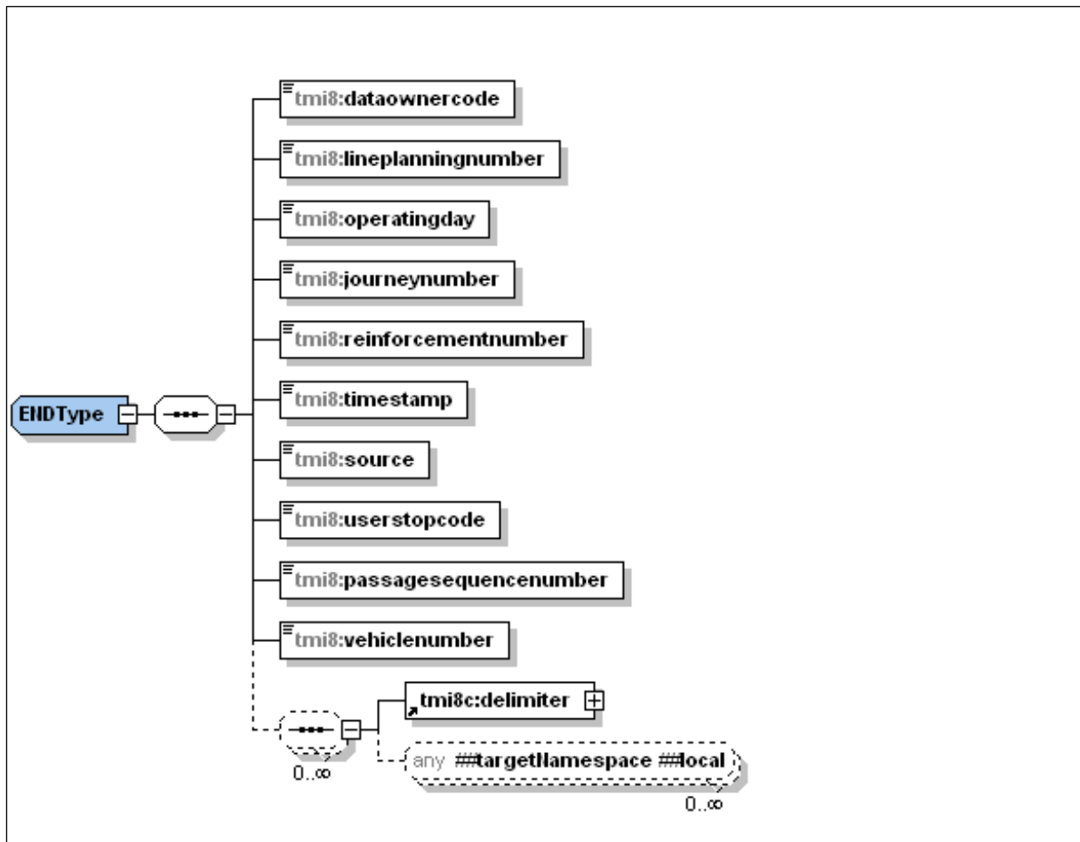
Figuur 30 XSD END
