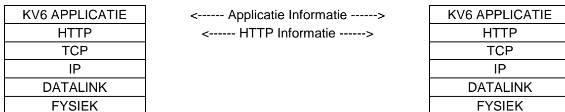
Figuur 31 koppelvlak protocol stapel
