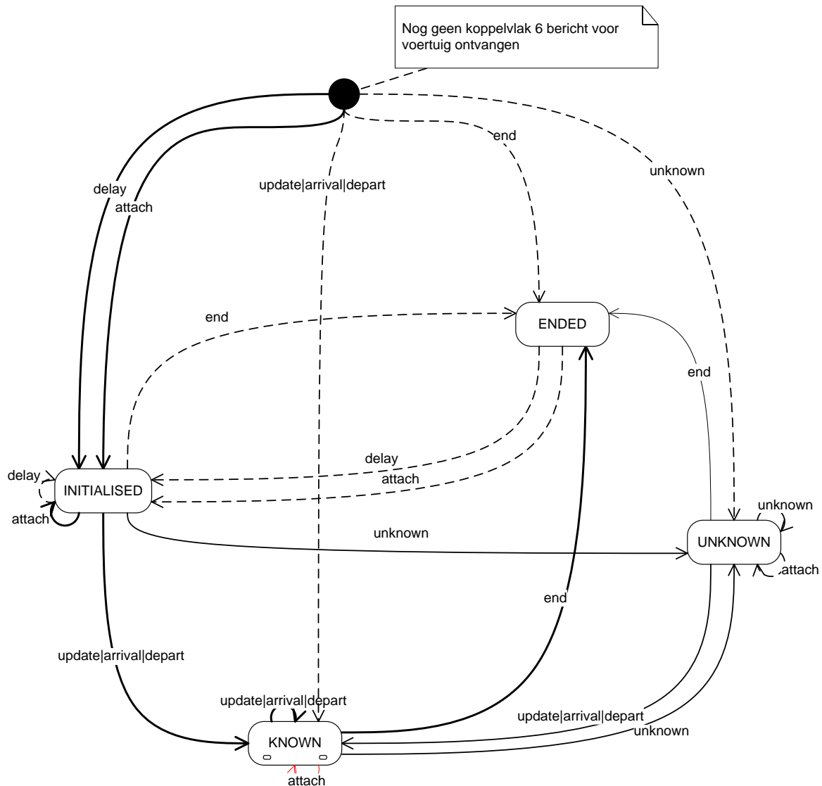
Figuur 37 Transitiediagram koppelvlak 6 berichten
