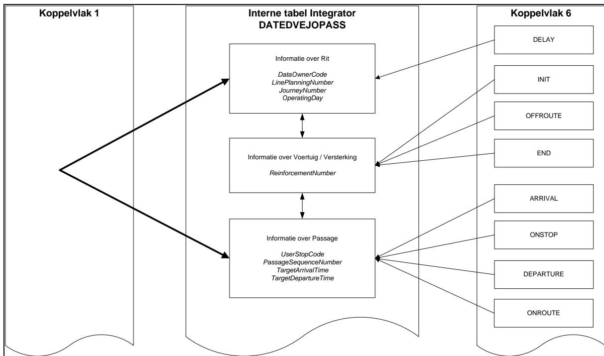
Figuur 33 Gebruik van DATEDVEJOPASS
