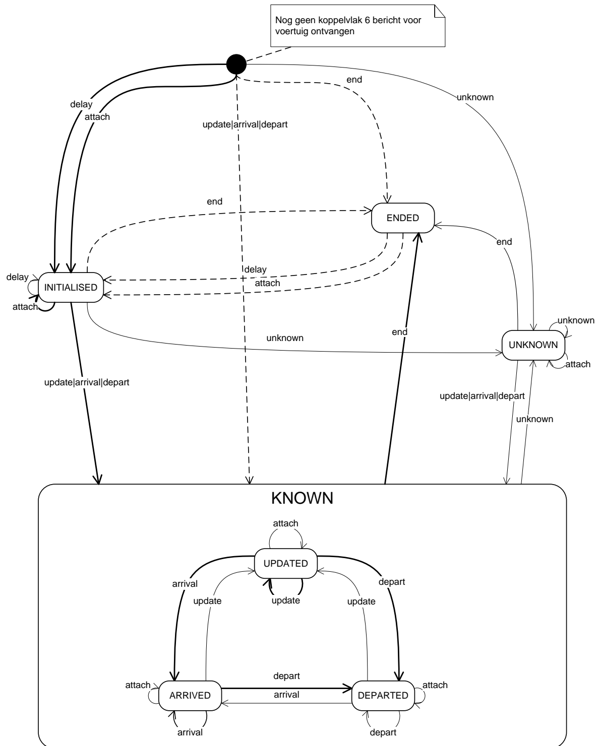
Figuur 38 Uitgebreid transitiediagram koppelvak 6 berichten
