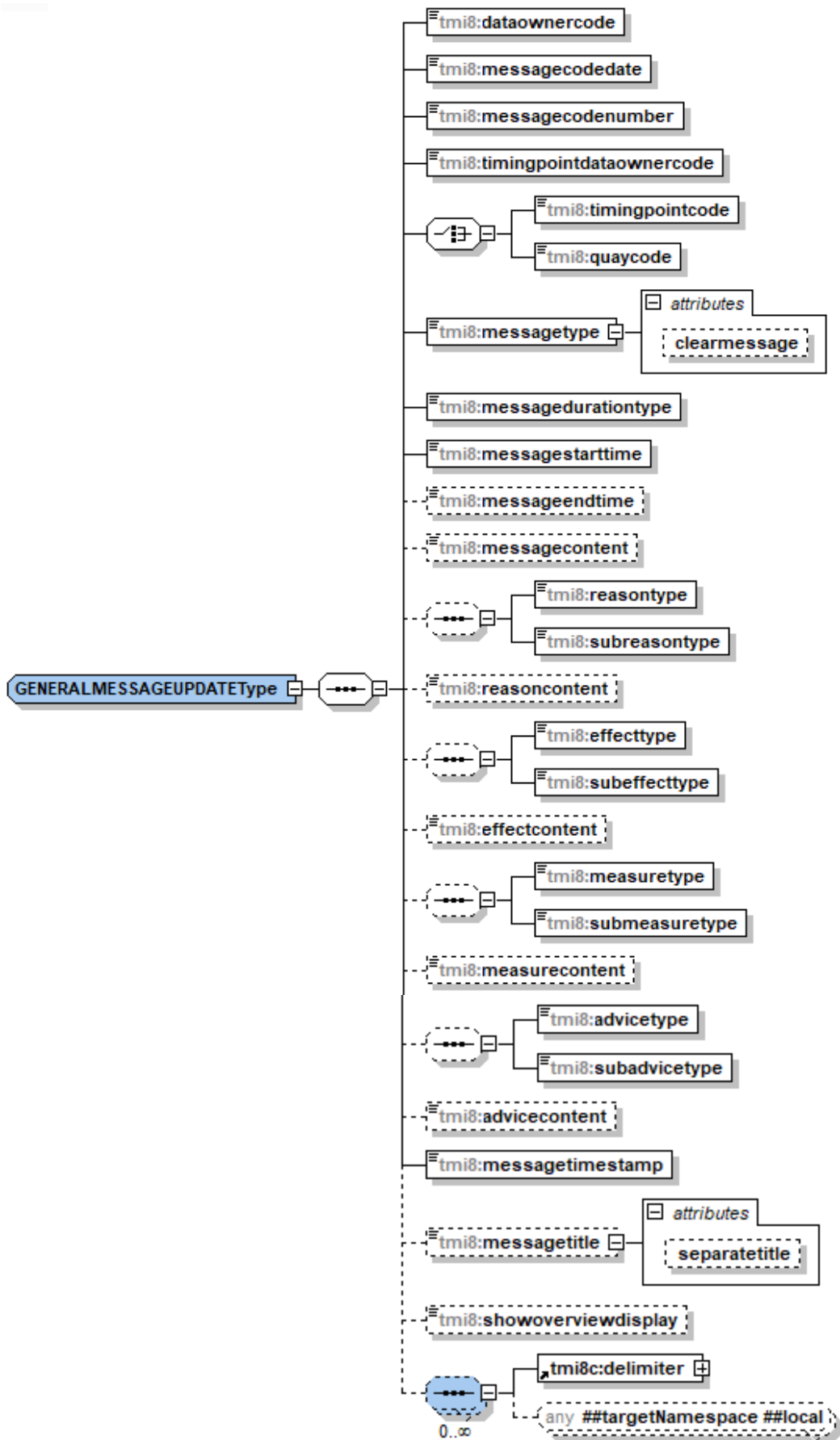
Figuur 32 XSD GENERALMESSAGEUPDATE
