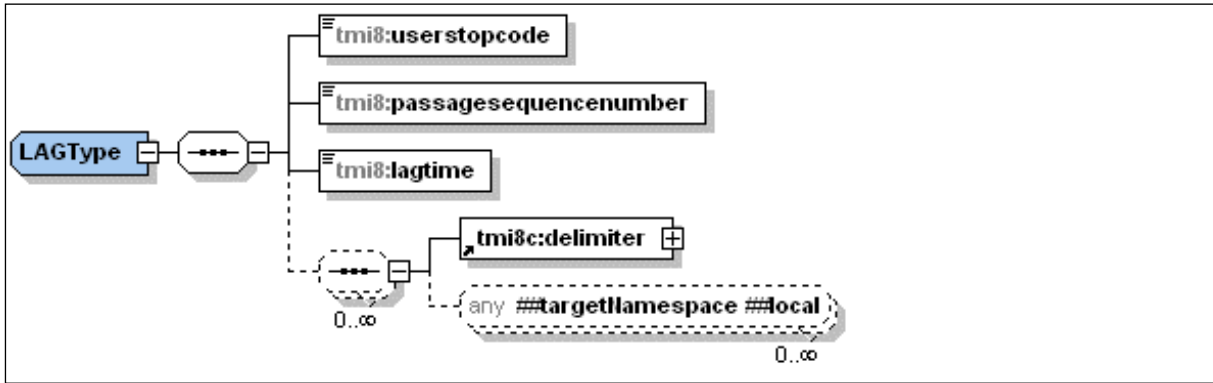
Figuur 20 XSD LAG
