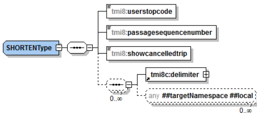
Figuur 19 XSD SHORTEN
