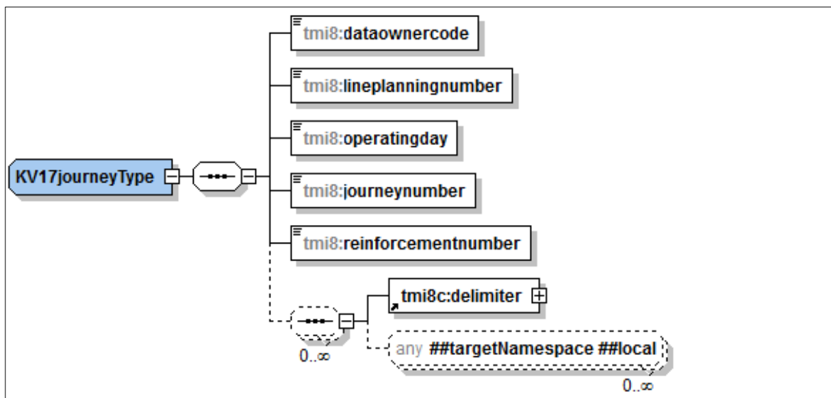
Figuur 14 XSD KV17JOURNEY
