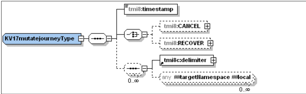
Figuur 15 XSD KV17MUTATEJOURNEY
