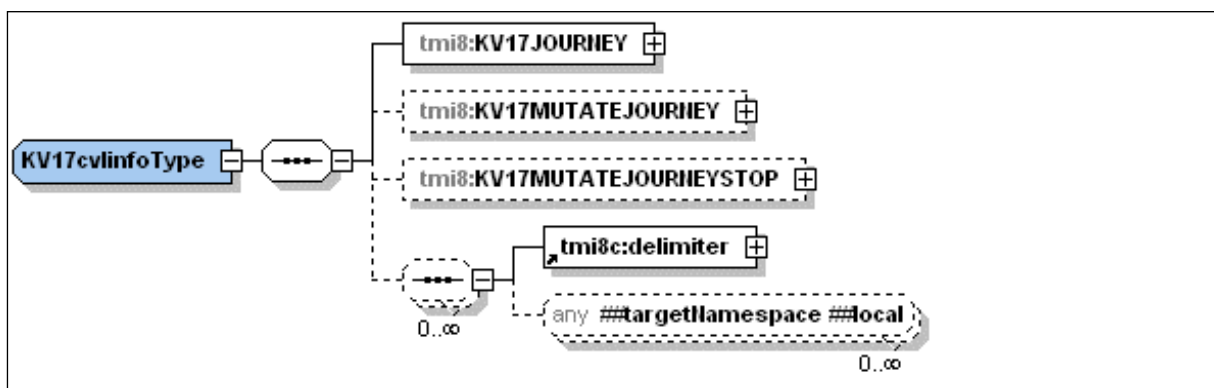
Figuur 13 XSD KV17cvlinfo
