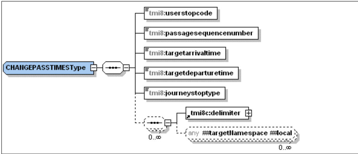
Figuur 21 XSD CHANGEPASSTIMES
