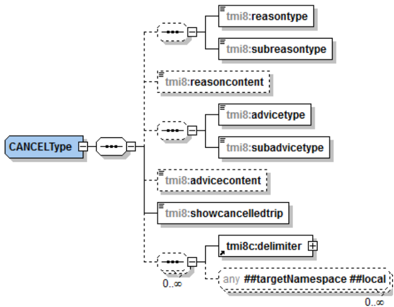
Figuur 17 XSD CANCEL
