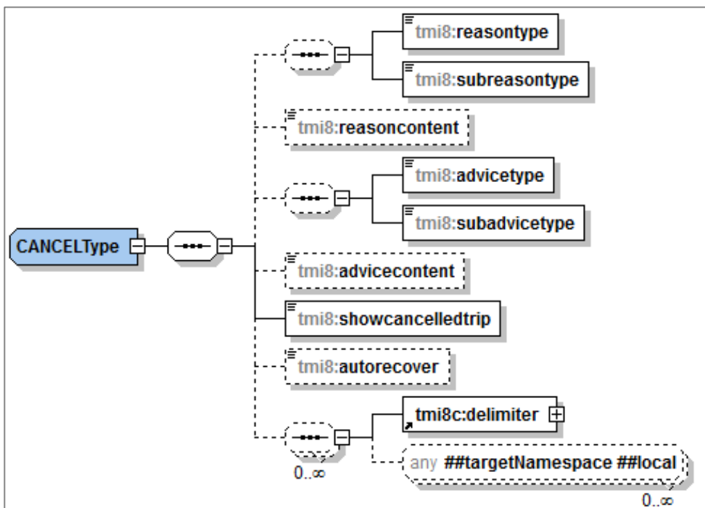
Figuur 17 XSD CANCEL
