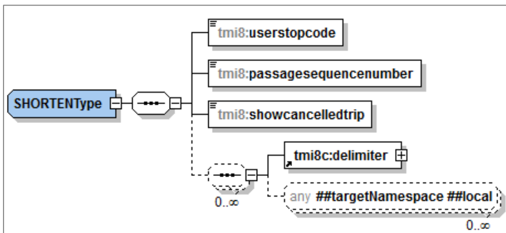
Figuur 20 XSD SHORTEN
