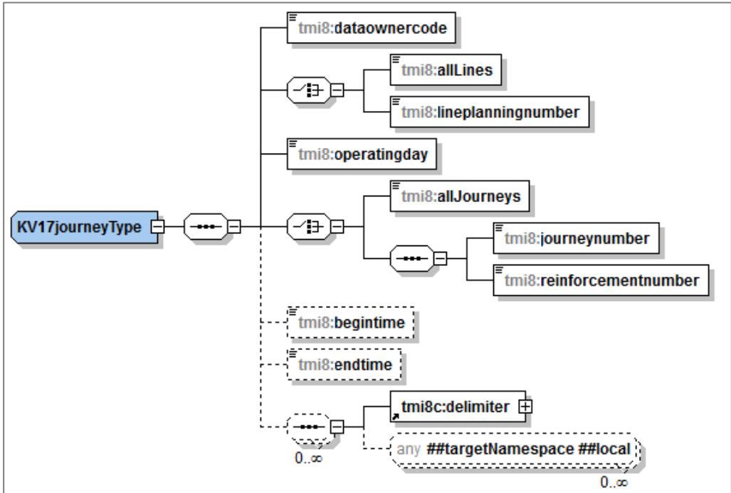
Figuur 14 XSD KV17JOURNEY
