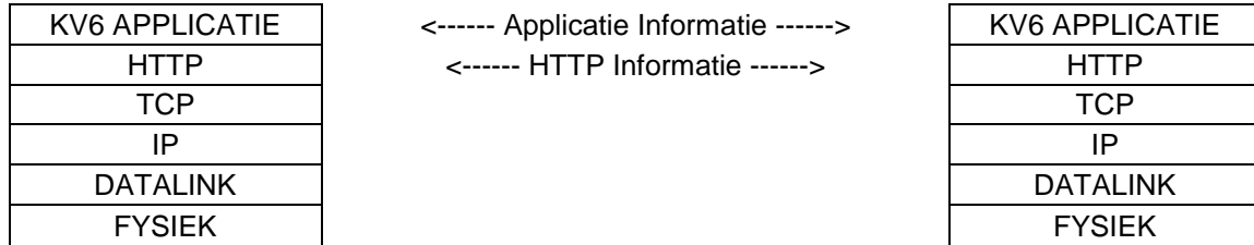
Figuur 31 koppelvlak protocol stapel
