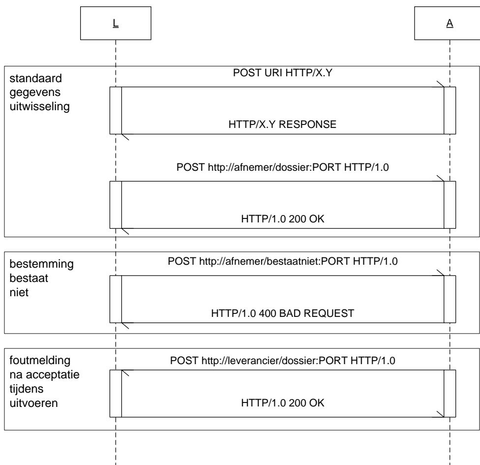
Figuur 2 HTTP POST protocol berichten uitwisseling (PORT is optioneel)
