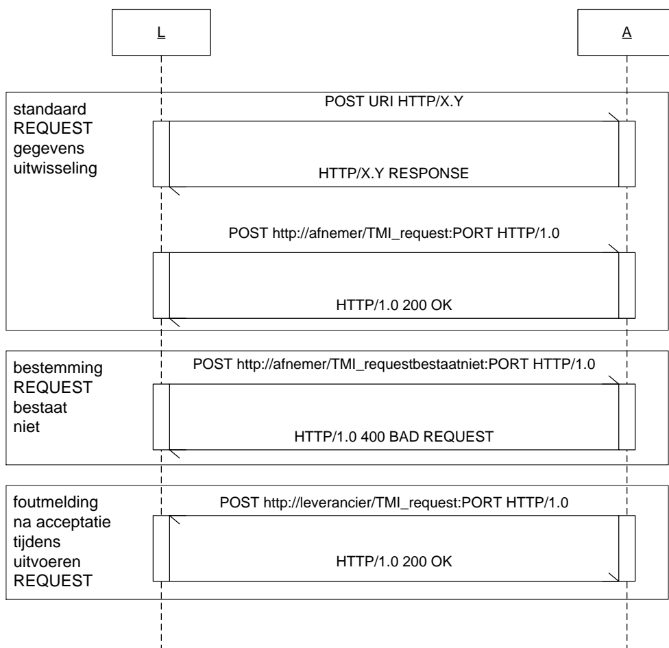
Figuur 3 HTTP REQUEST protocol berichten uitwisseling (PORT is optioneel)
