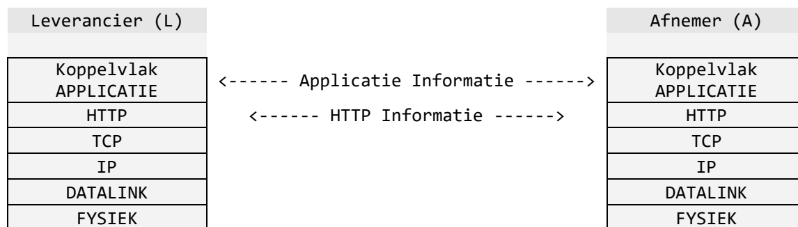
Figuur 1 koppelvlak protocol stapel
